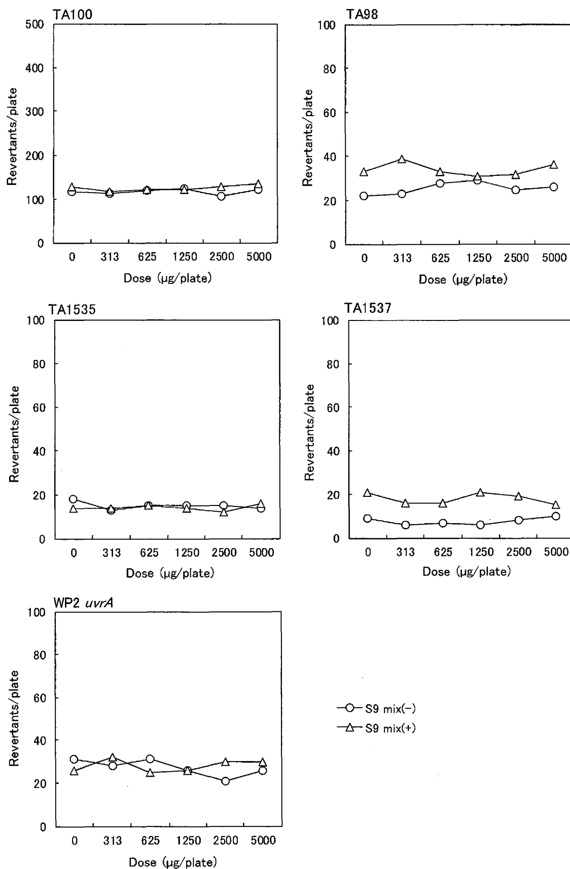
図 2 1-Ethoxy-2-(2-methoxyethoxy)ethane の細菌を用いる復帰突然変異試験(本試験 II)
