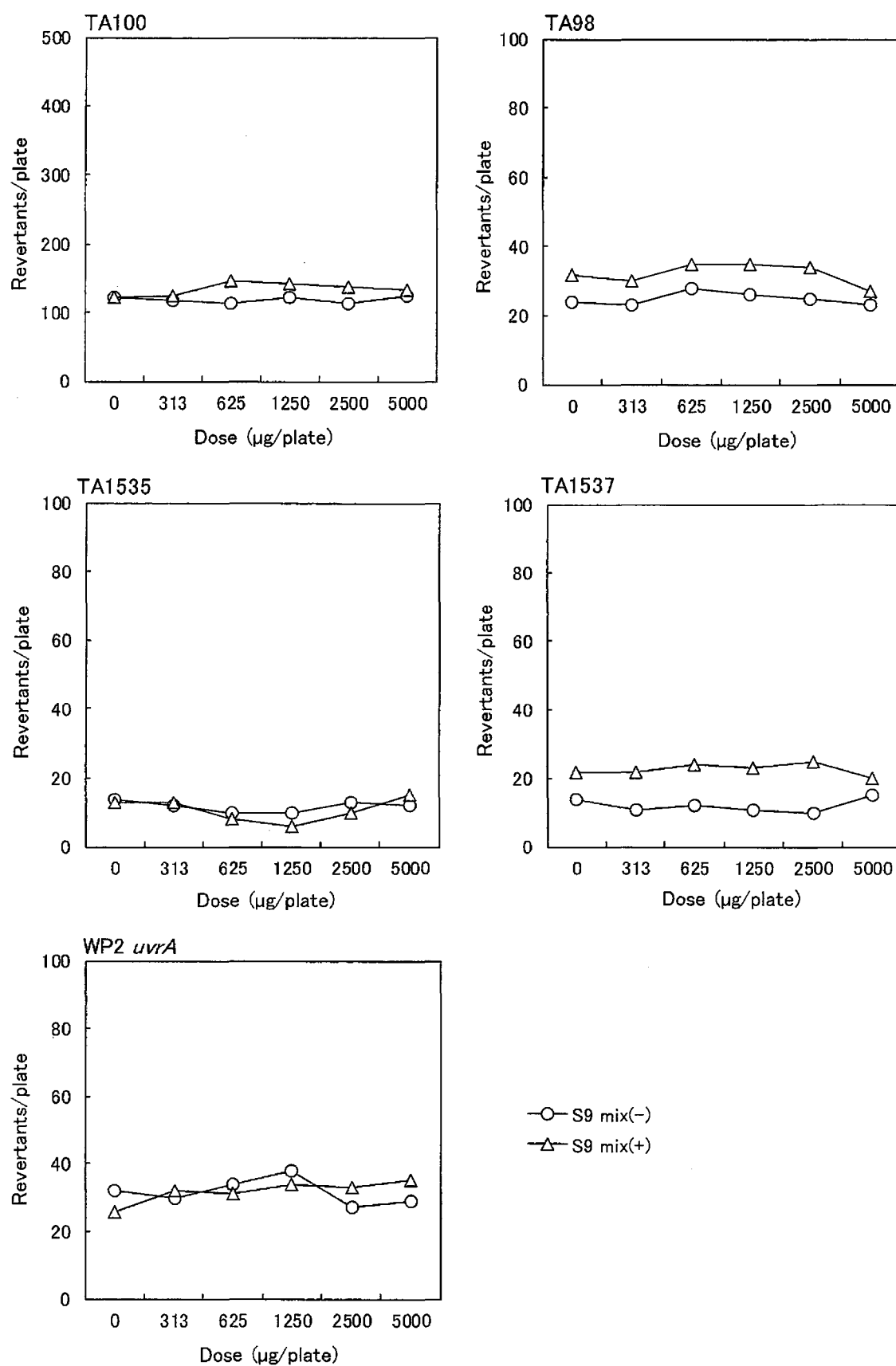
図 1 1-Ethoxy-2-(2-methoxyethoxy)ethane の細菌を用いる復帰突然変異試験(本試験 I)
